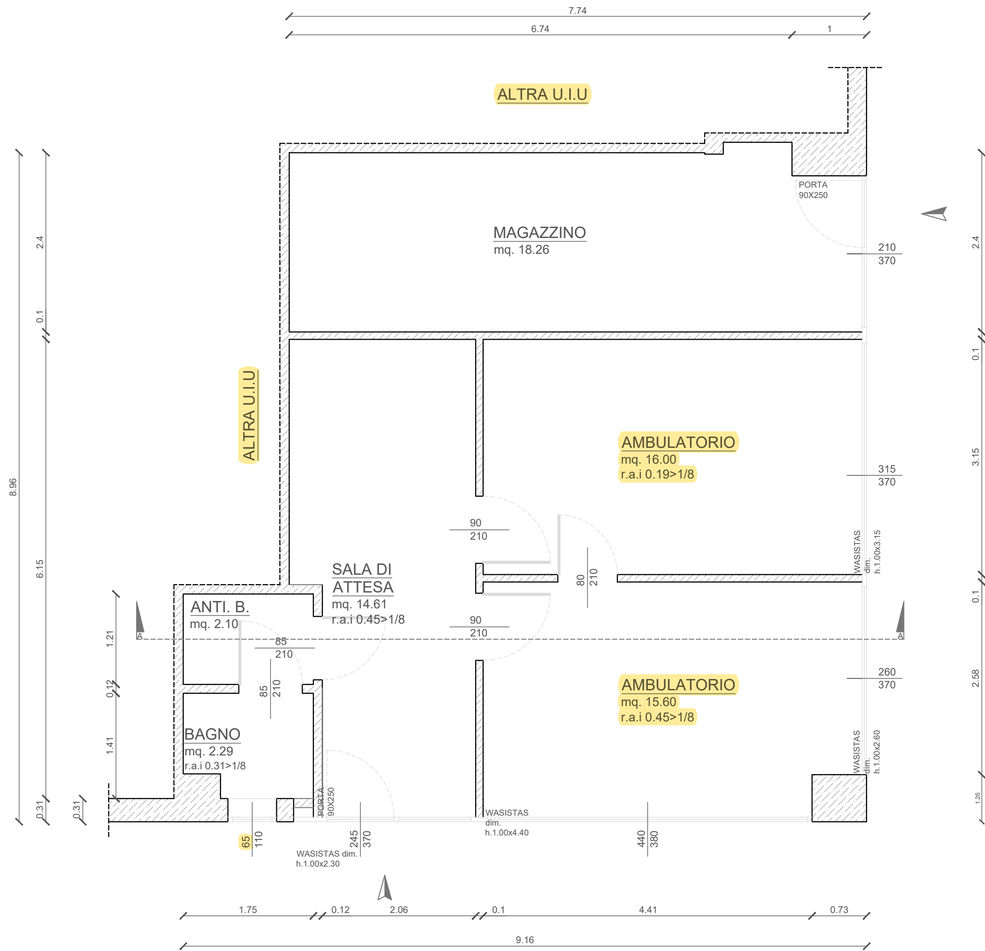
PIANO TERRA scala 1:50
